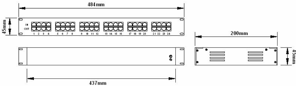
Рис.2 Габаритные размеры SP-IP8(16,24)/100(1000)
