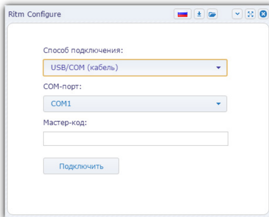
Рисунок 4. Настройка USB-соединения в программе Ritm Configure
