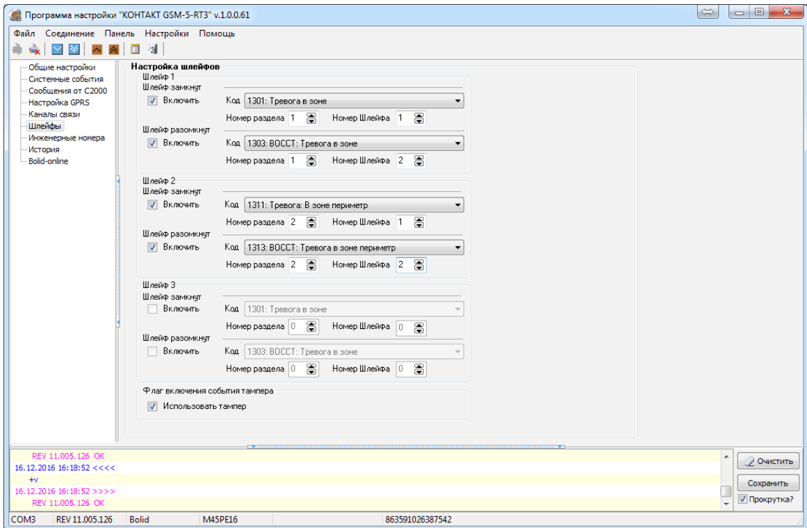
Рисунок 21. Настройки шлейфов: шлейфы типа «сухой контакт»
