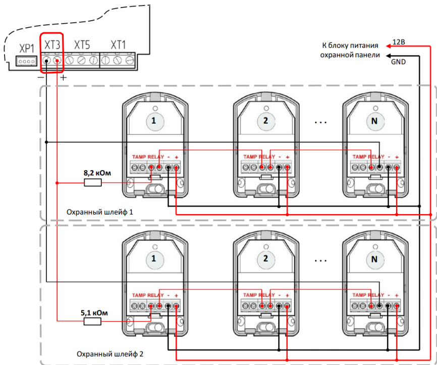
Рисунок 37. Схема подключения резистивных шлейфов
