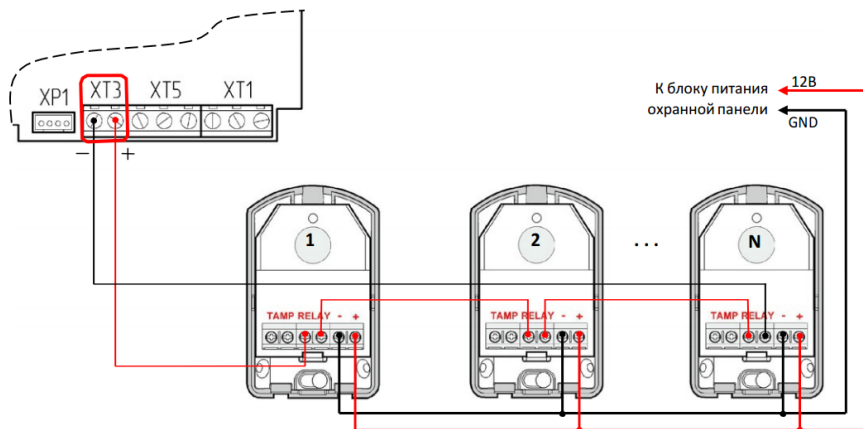
Рисунок 36. Схема подключения датчиков «сухие контакты»
