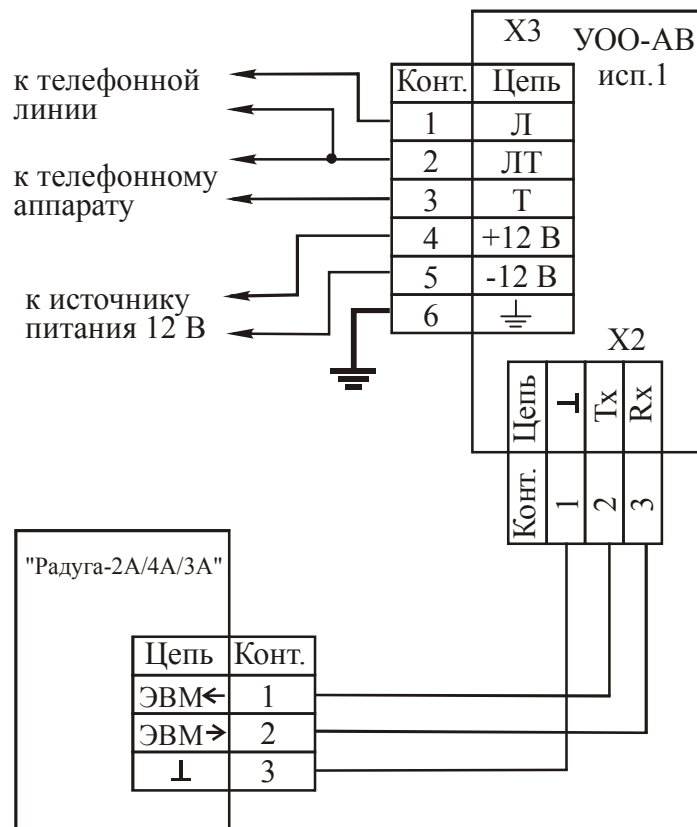
Схема внешних подключений УОО-АВ исполнения 1 при работе с ППКП "Радуга-2А", "Радуга-4А", "Радуга-3"
