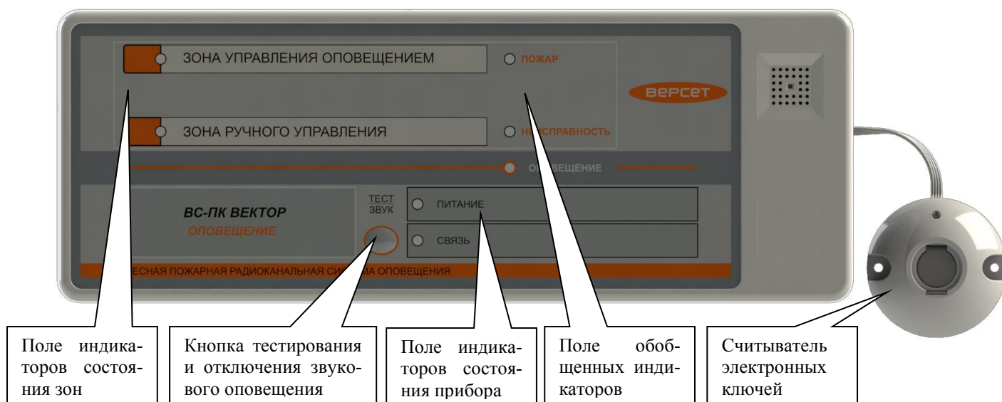
Рис.1 Внешний вид прибора
