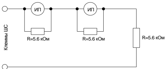
Схема включения пожарных извещателей со стратегией Тепловой
