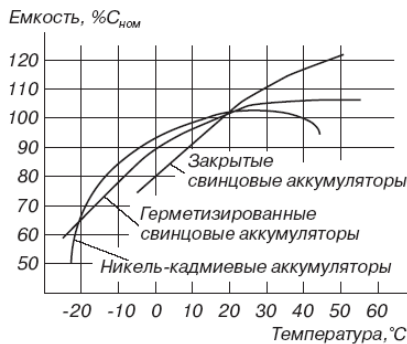
Рис. 5. Зависимость ёмкости АКБ от температуры
