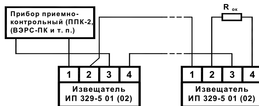
Пример схемы подключения извещателей ИП 329-5 01 и ИП 329-5 02 к двухпроводной системе пожарной сигнализации
