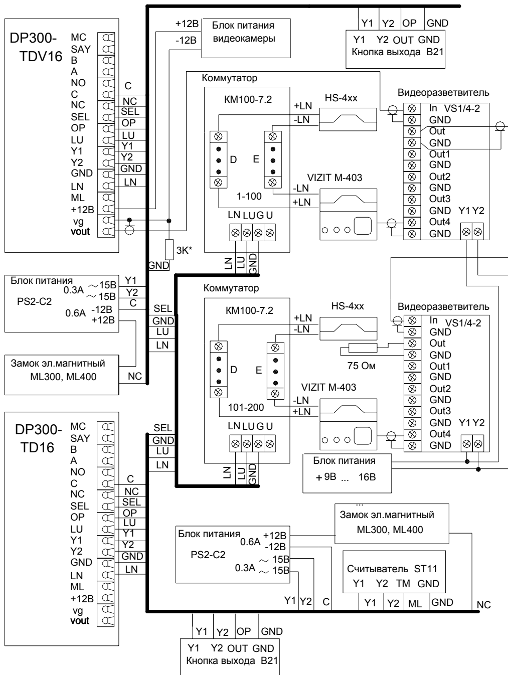
Рис.3 Пример схемы подключения DP300-TDV16 в составе домофонного комплекса.
