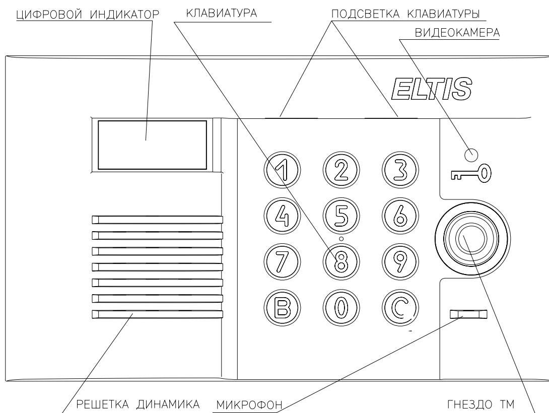
Рис.1 Внешний вид со стороны лицевой панели блока вызова DP300-TDV16.
