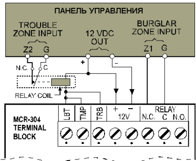
Рисунок 7. Подключение всех контактов статуса к одной Н.З. зоне
