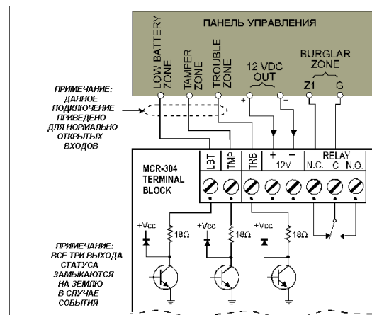
Рисунок 5. Общая схема подключения
