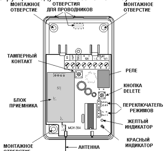
Рисунок 2. MCR-304 со снятой крышкой
