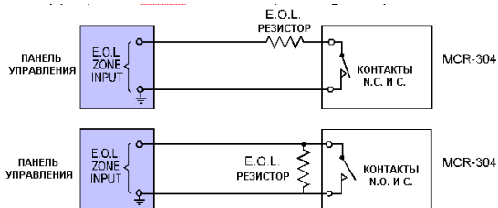
Рисунок 4. Подключение E.O.L. резистора к релейному выходу
