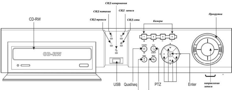
Вид панели регистратора.
