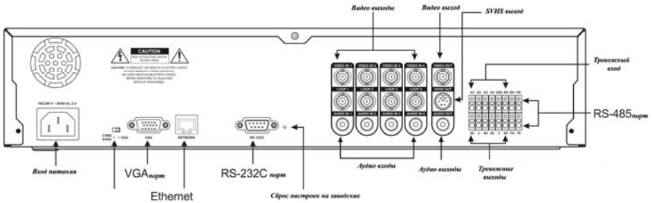
Задняя панель регистратора.
