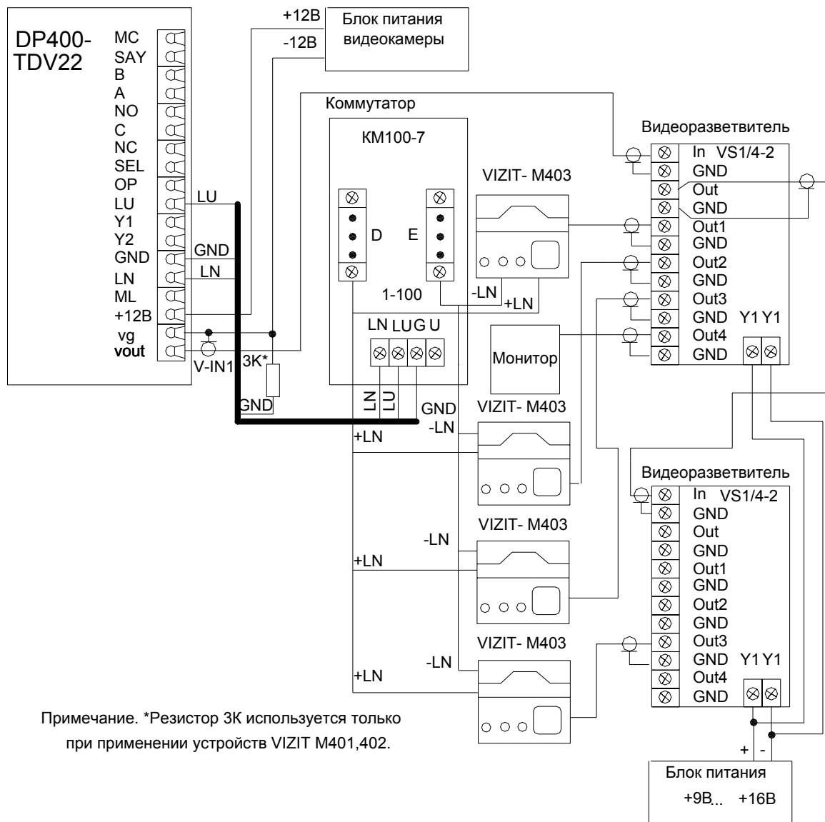
Рис.5 Схема подключения видеоканала блока вызова DP400-TDV22. (Пример с двумя видеоразветвителями)
