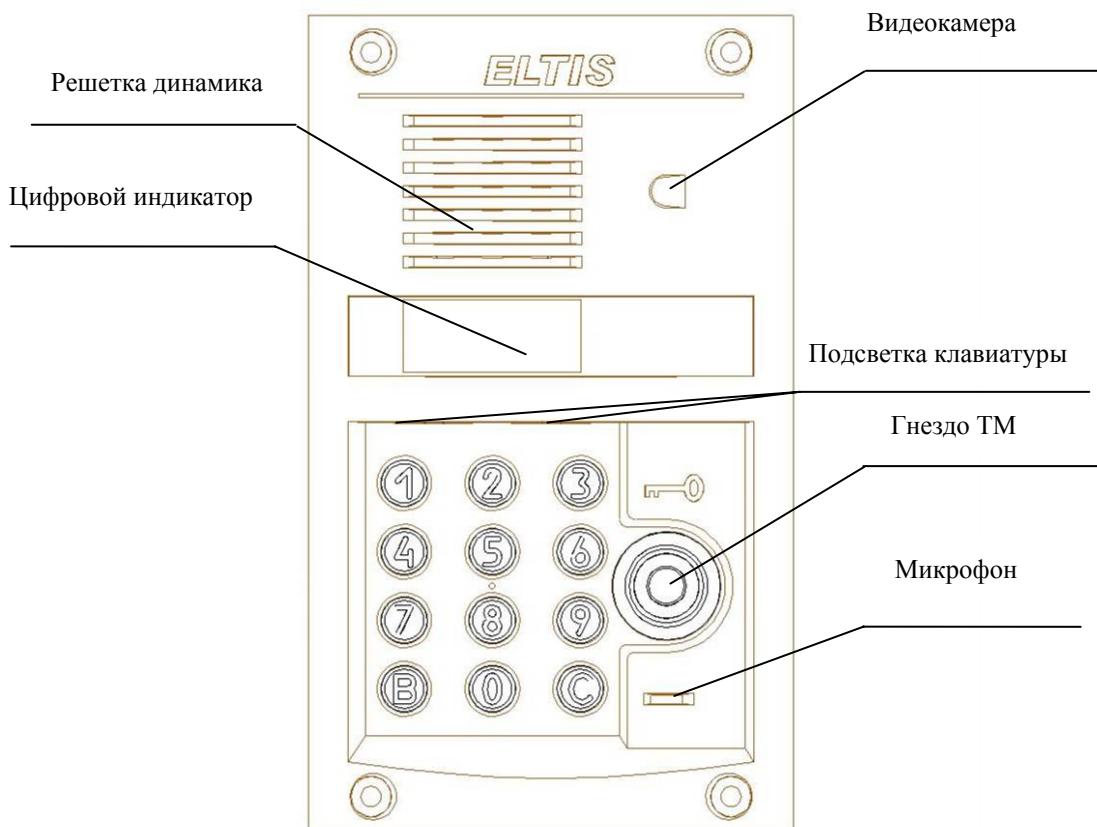
Рис.1 Внешний вид со стороны лицевой панели блока вызова DP400-TDV22.
