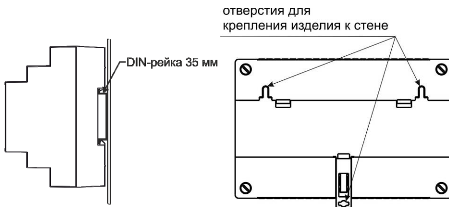
Рисунок 1 - крепление изделия
