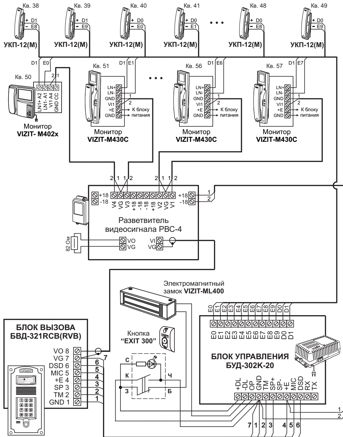
Рисунок 6 - Пример схемы соединений видеодомофона с использованием блока управления БУД-302К-20 и блока вызова БД-321RCB(RVB)
